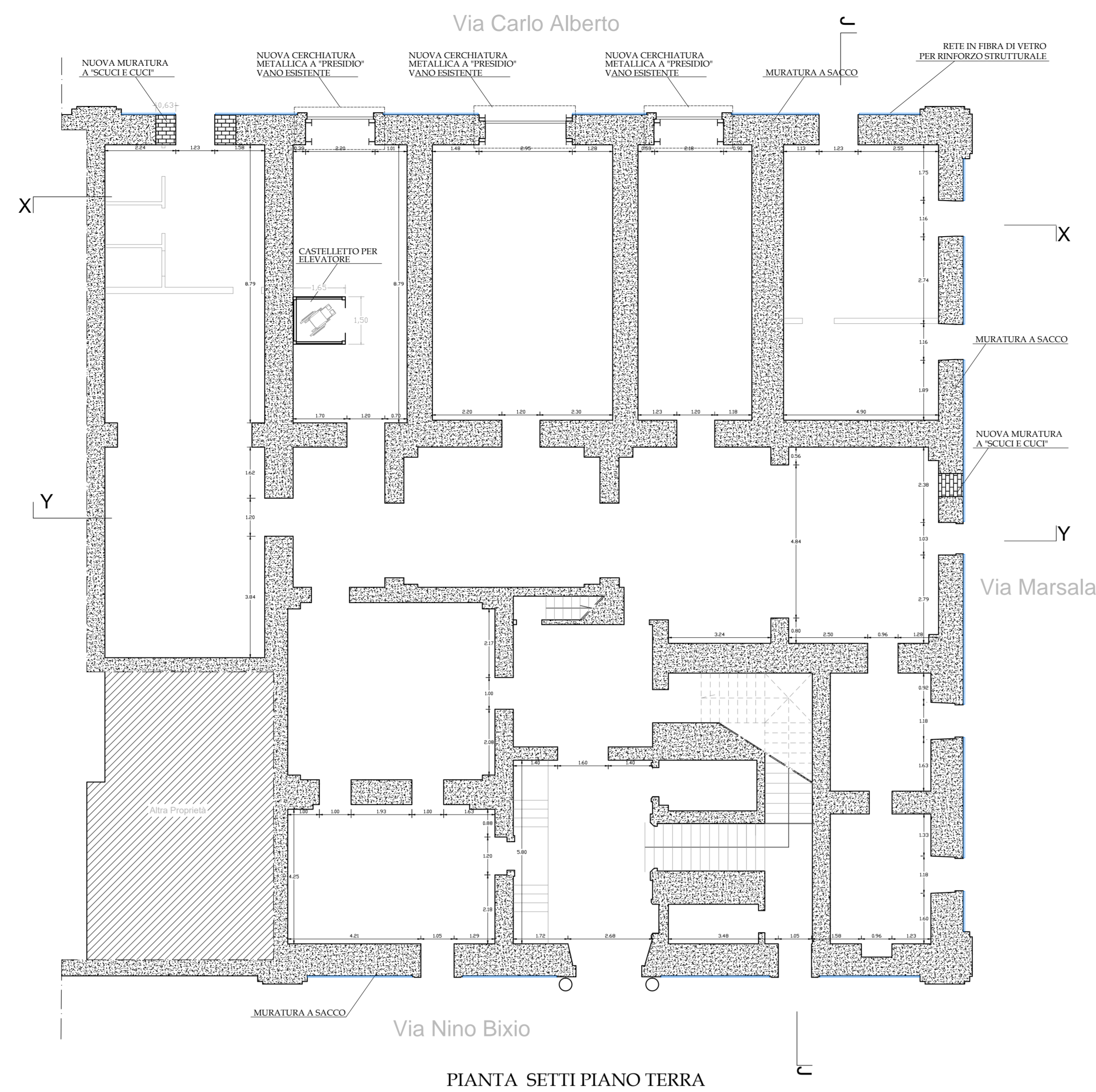
PIANTA SETTI PIANO TERRA
