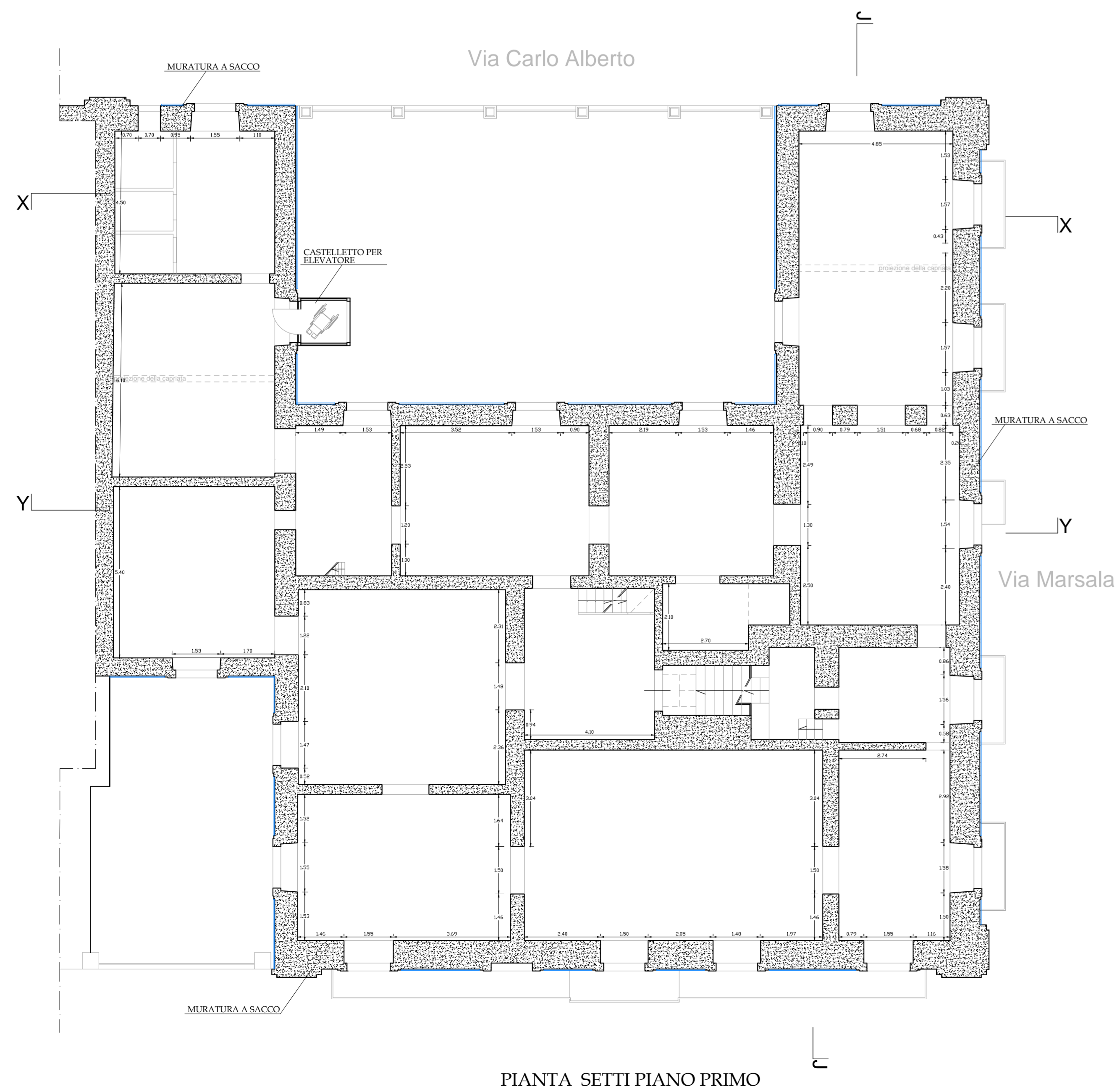
PIANTA SETTI PIANO PRIMO
