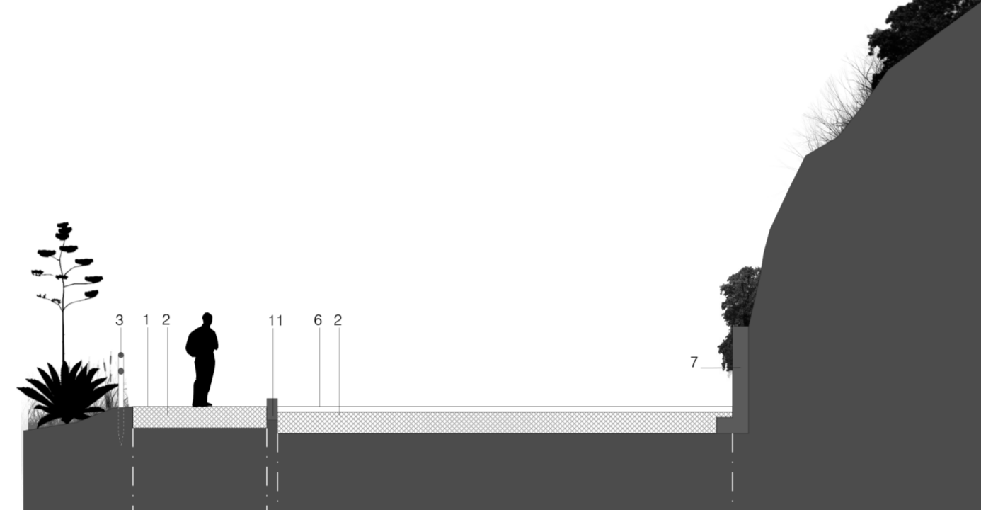
sezione tipo 12 1:100
