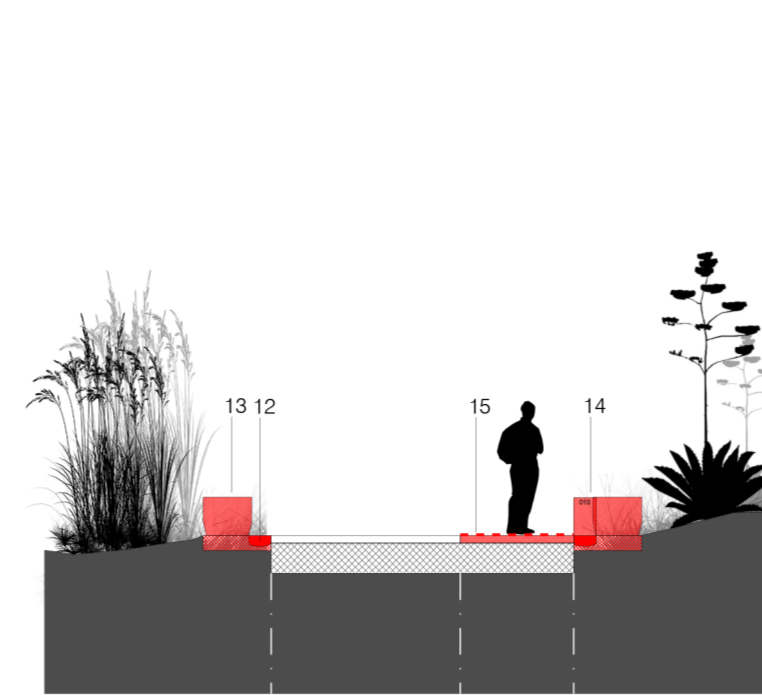
sezione tipo 14 progetto 1:100
