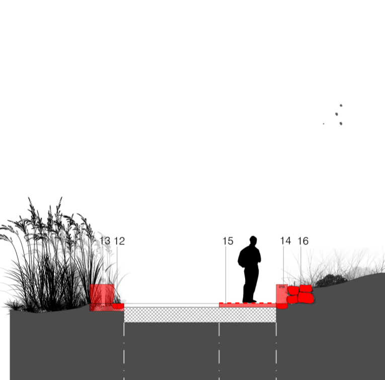
sezione tipo 11 progetto 1:100
