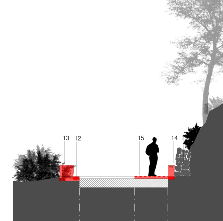
sezione tipo 15 progetto 1:100
