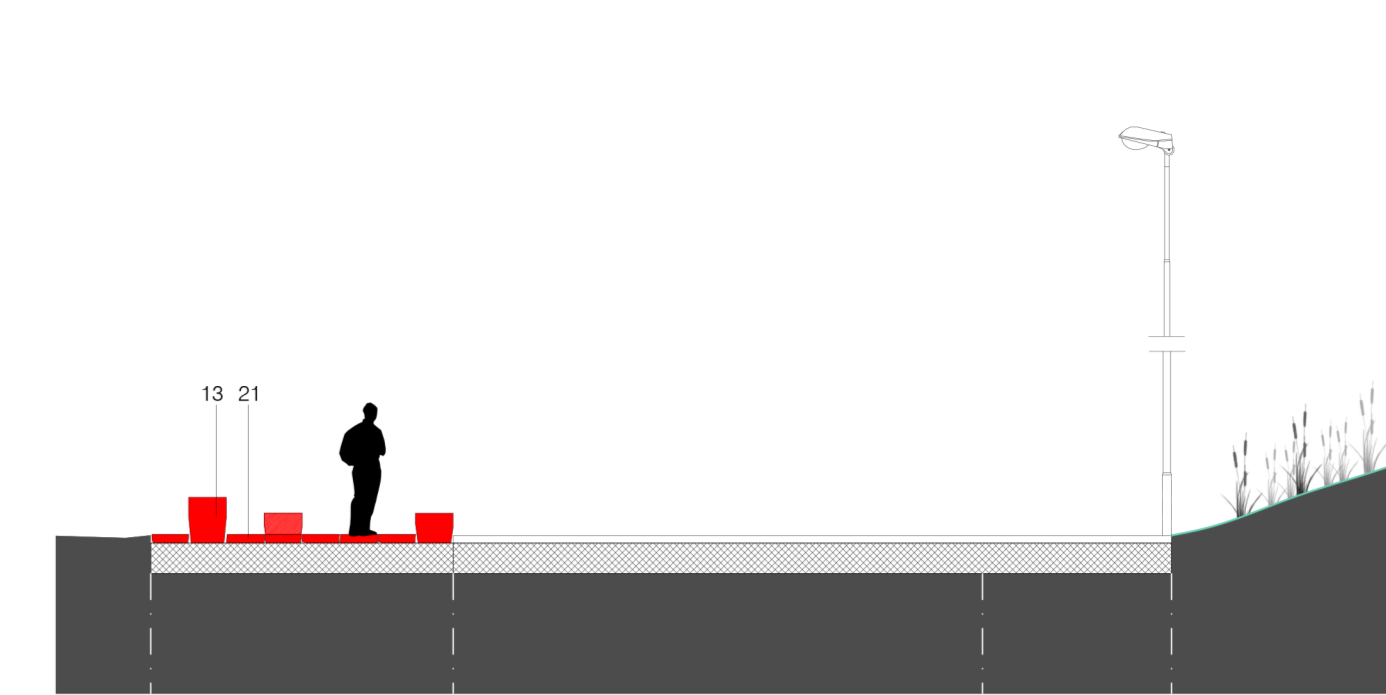
sezione tipo 18 progetto 1:100
