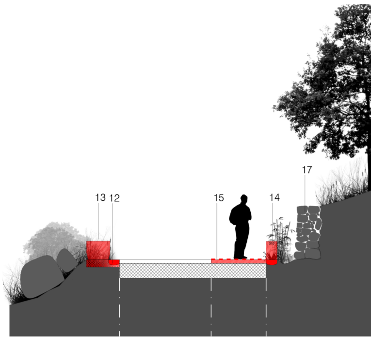
sezione tipo 10 progetto 1:100
