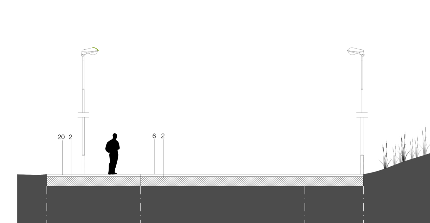
sezione tipo 18 1:100
