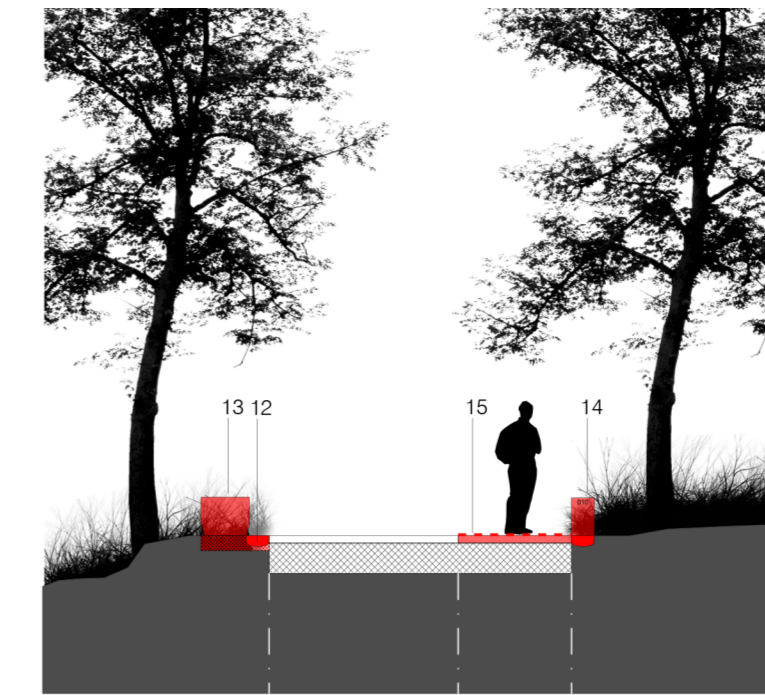
sezione tipo 16 progetto 1:100
