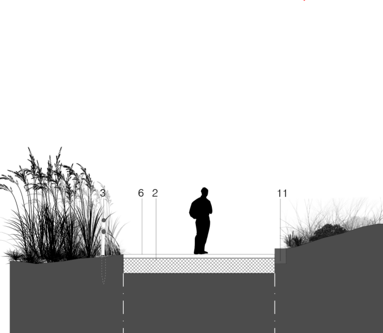
sezione tipo 11 1:100
