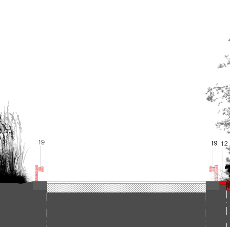
sezione tipo 16 1:100
