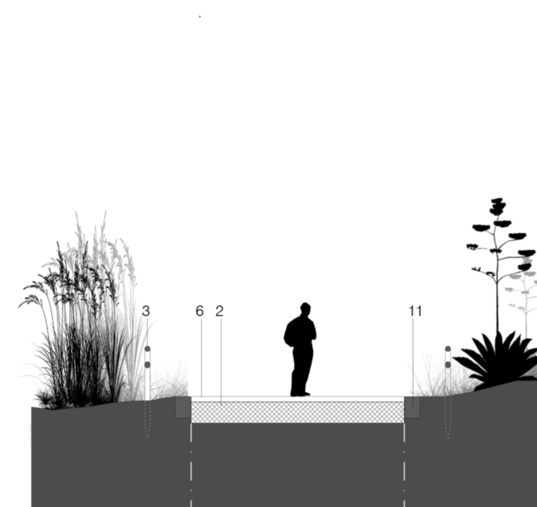
sezione tipo 14 1:100
