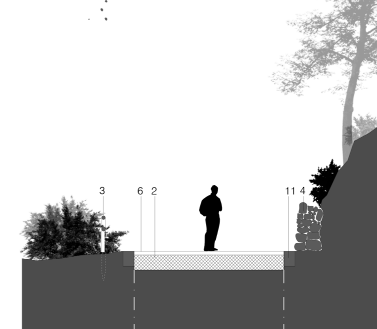
sezione tipo 15 1:100
