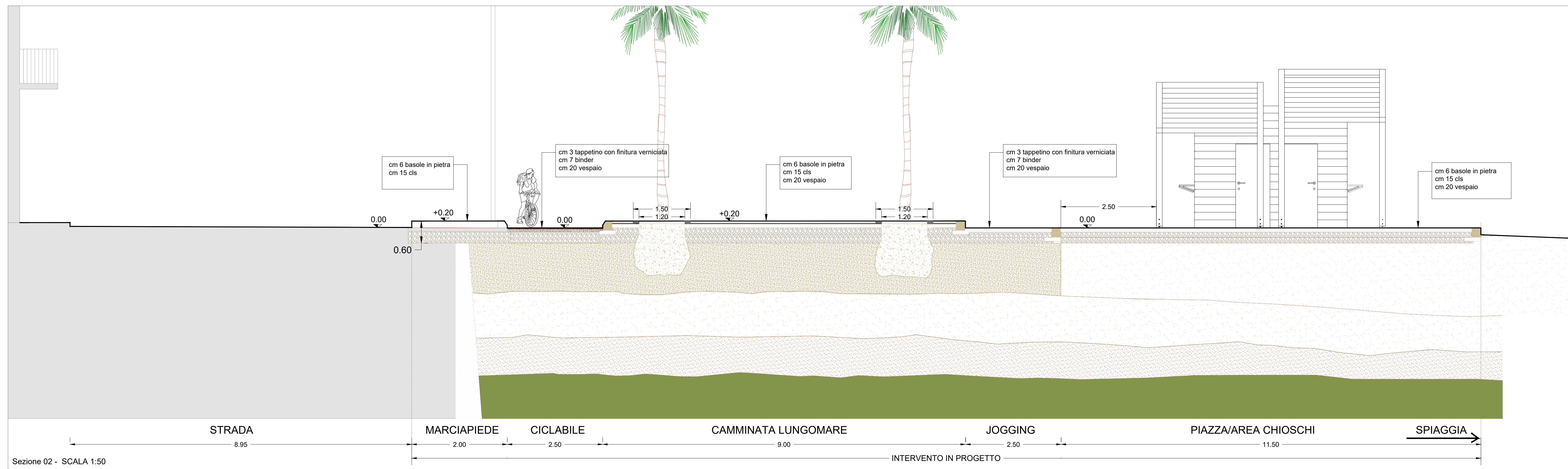
Sezione 02 - SCALA 1:50
