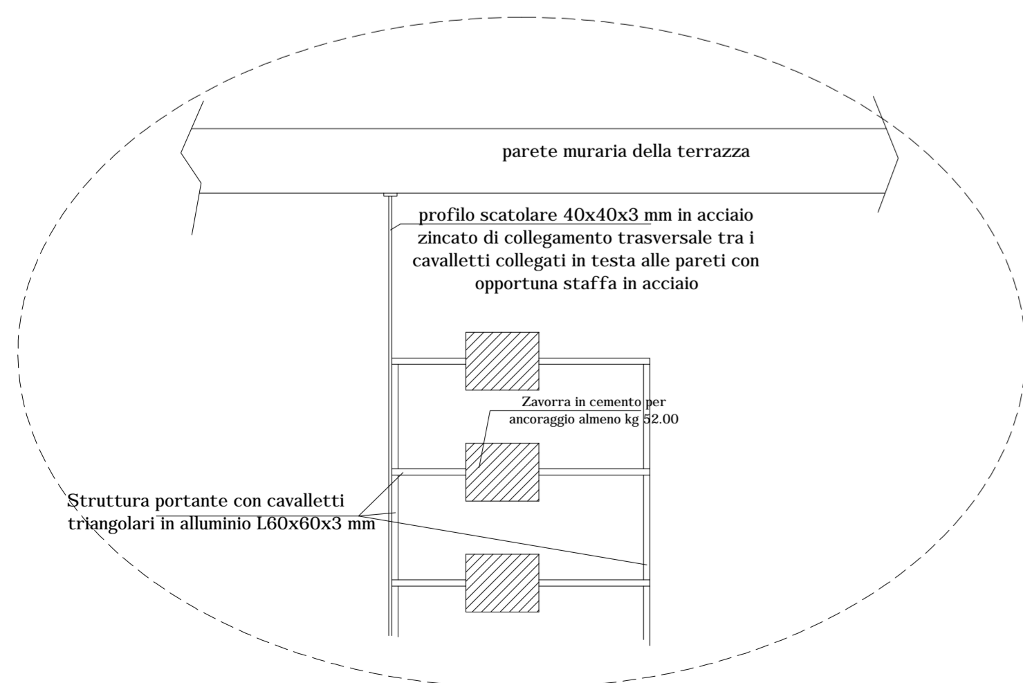
PARTICOLARE STRUTTURA FOTOVOLTAICO
