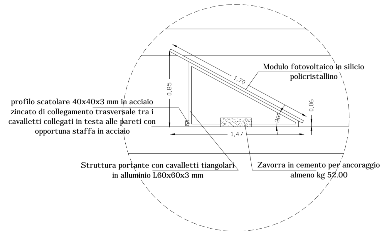
PARTICOLARE STRUTTURA FOTOVOLTAICO
