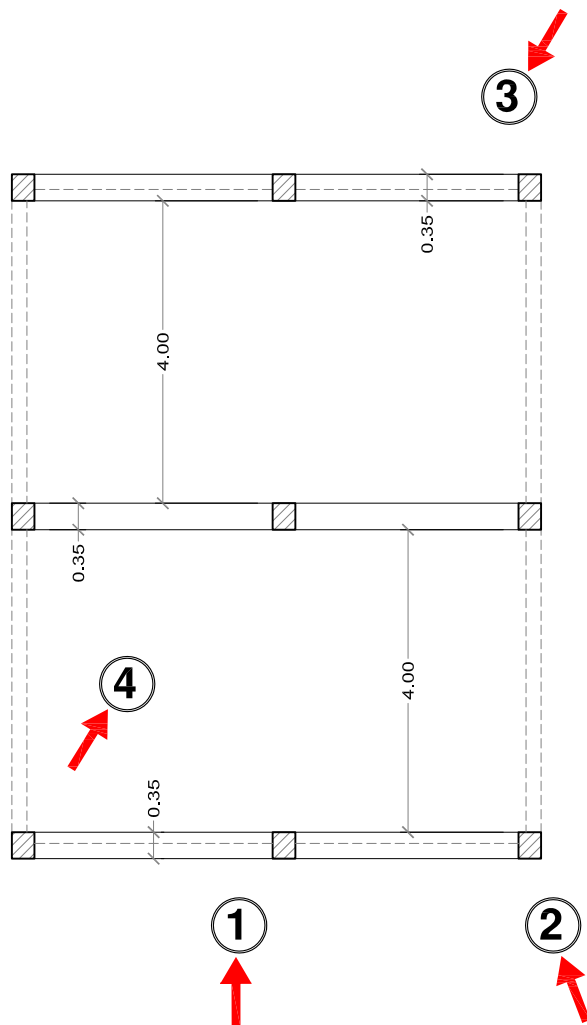
PIANTA Scala 1:100
