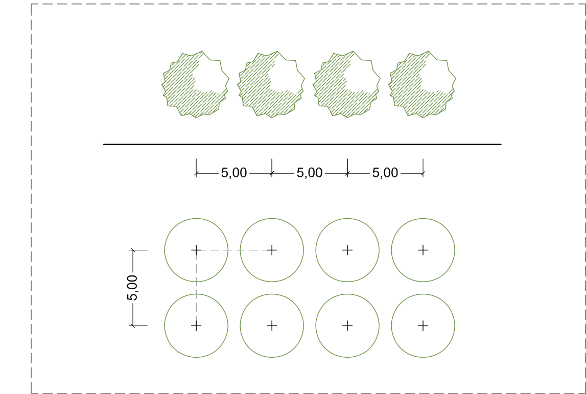
SCHEMA IMPIANTO DI FILARE SEMPLICE PER AREE DI PARCHEGGIO
