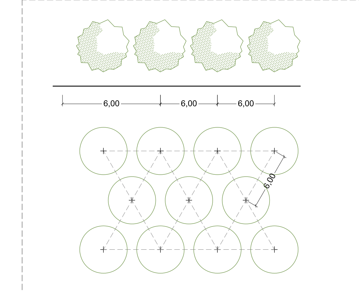
SCHEMA IMPIANTO ARBOREO A SESTO REGOLARE PER BARRIERE ARBOREE
