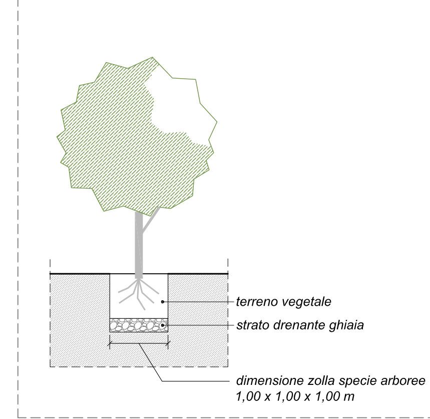
SEZIONE TIPO IMPIANTO SPECIE ARBOREE
