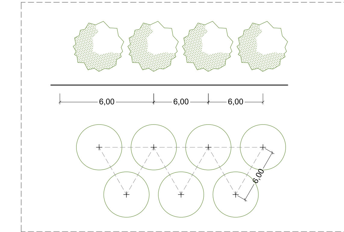
SCHEMA IMPIANTO DI FILARE COMPOSTO PER BARRIERE ARBOREE
